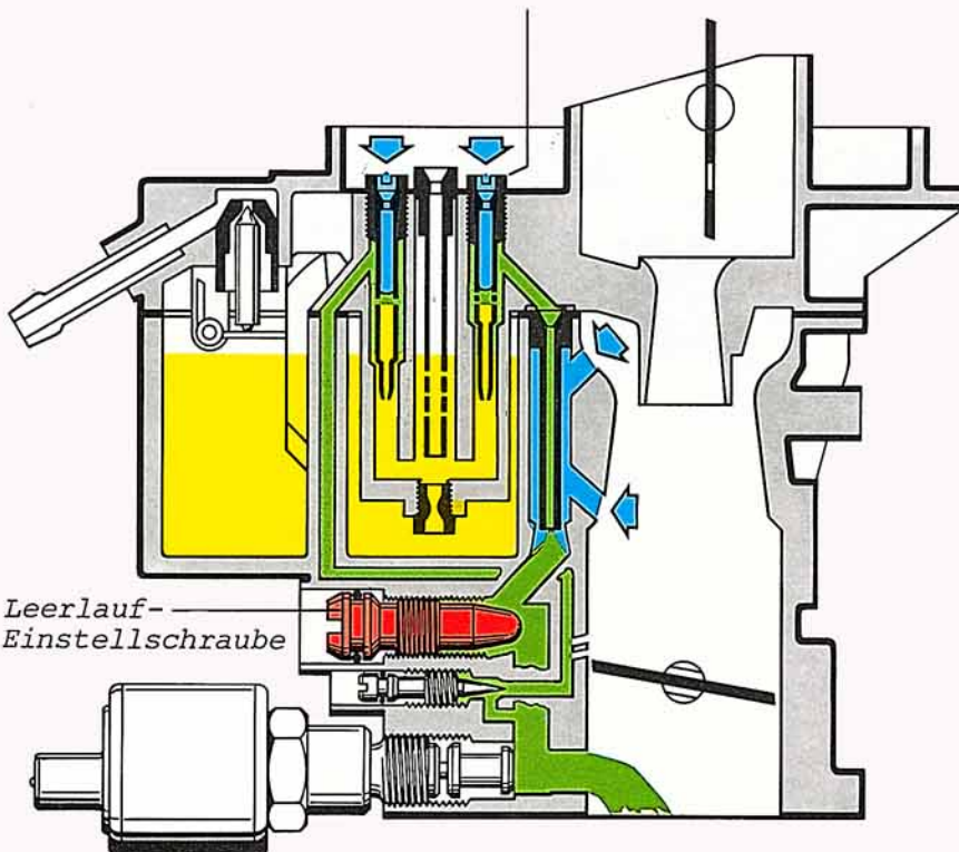
Zusatz-Kraftstoff-Luftdüse
