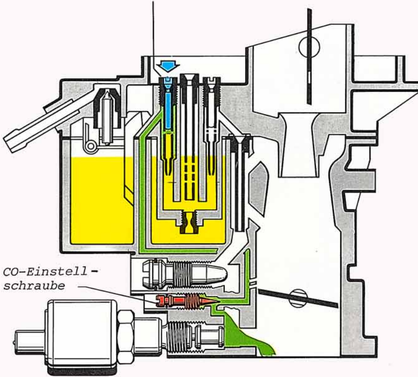
Leerlauf-Kraftstoff-Luftdüse
