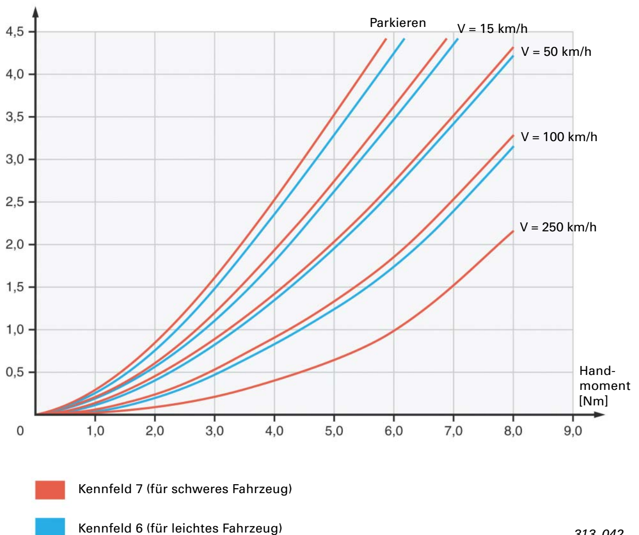
V187-Motormoment [Nm]
