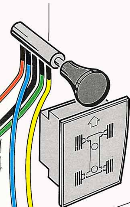
Zweistufiger Schalter Er steuert den Druck für die Schaltelemente.
