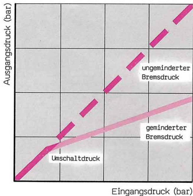
Regler-Kennlinie
