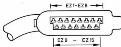
Zentralstecker VEZ-Steuergerät
