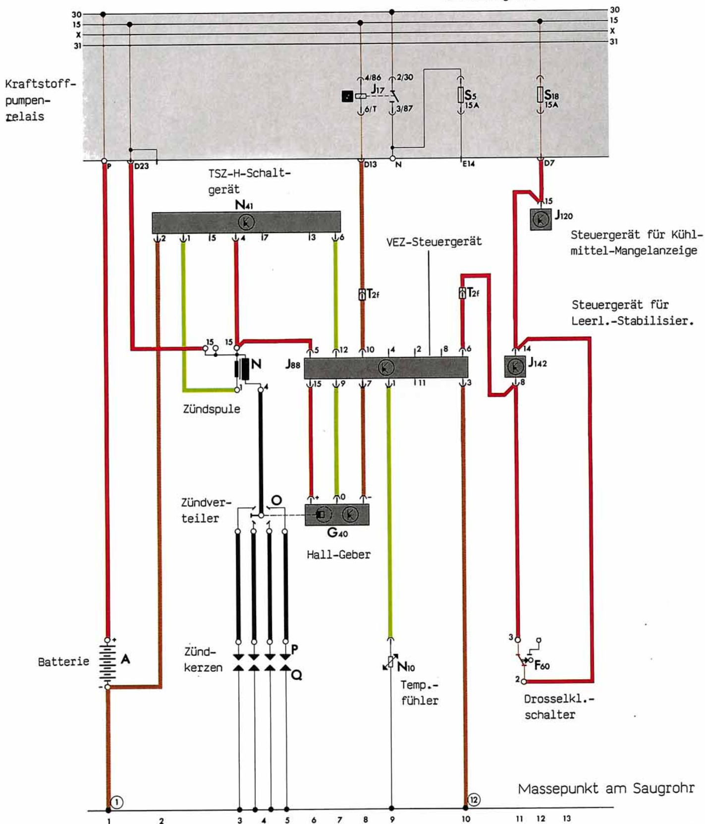
Zentralstecker VEZ-Steuergerät
