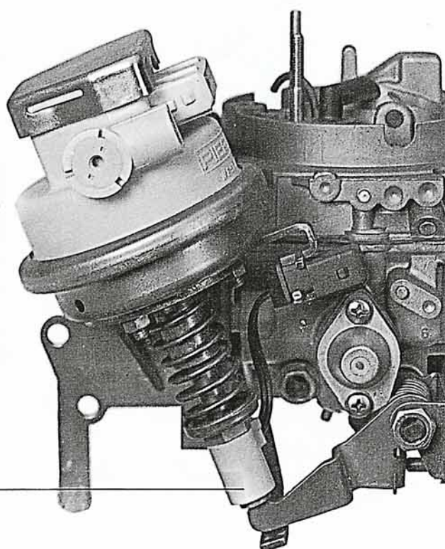
Leerlaufschalter, im Leerlauf geöffnet
