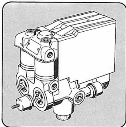
Hydraulikeinheit
