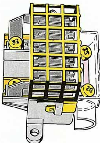
J52 Relais für Glühkerzen
