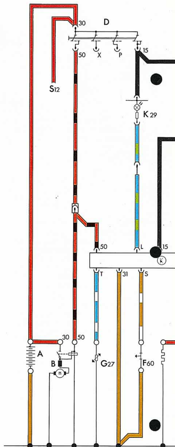
G27 Geber für Motortemperatur
